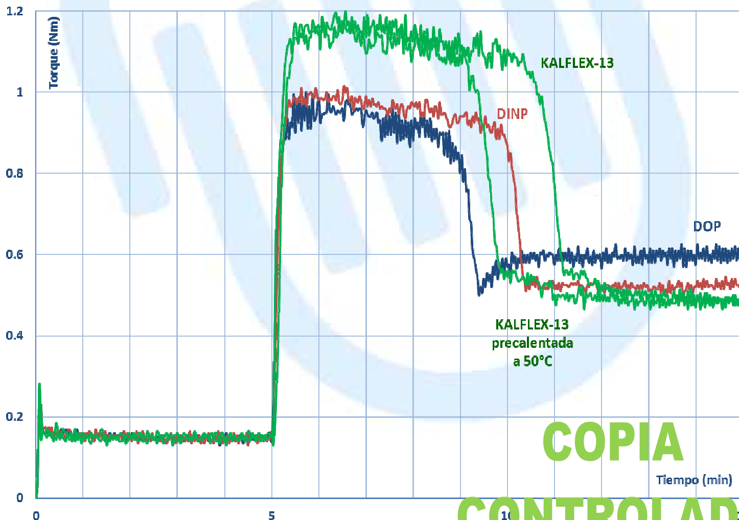
CURVA DE ABSORCIÓN CON RESINA DE SUSPENSIÓN
